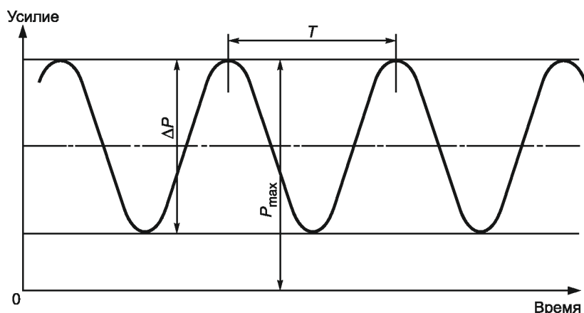
Рисунок Е.1 — Обозначения параметров повторяющейся нагрузки
